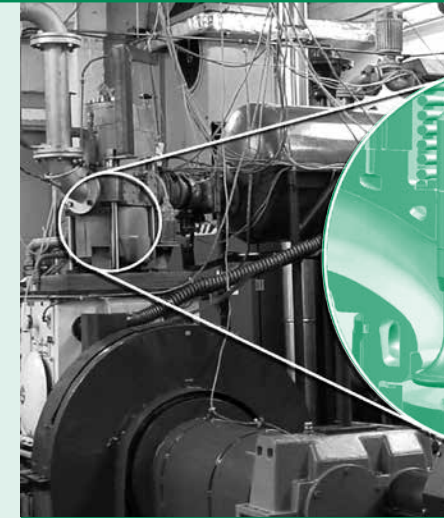
Zweistoffbetrieb an einem Dieselmotor
