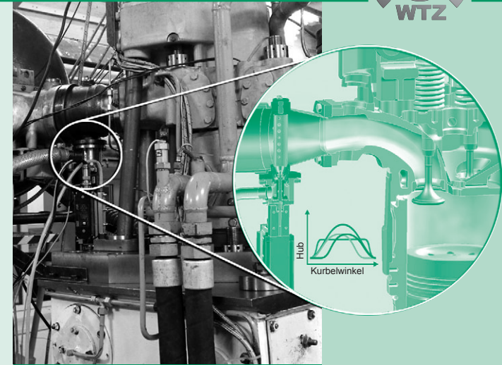
Variables Gasventil in einem mittelschnelllaufenden Motor
